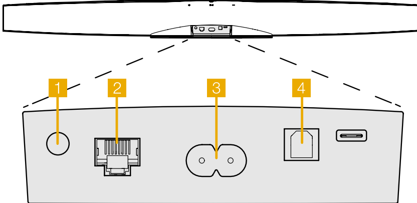
الشكل 1 اللوحة الخلفية لجهاز فورميشن بار
