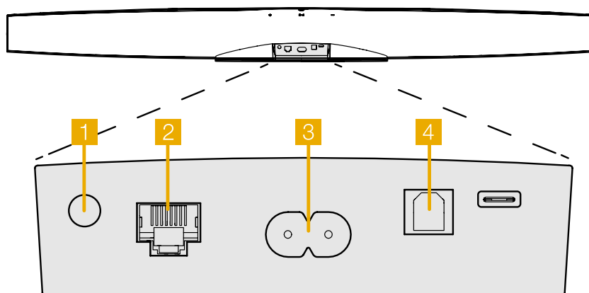
Διάγραμμα 1 Πίσω μέρος του Formation Bar
