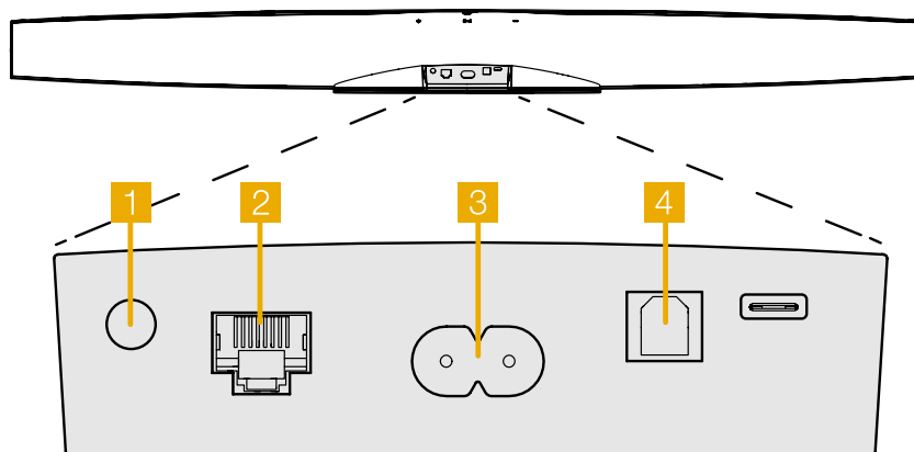
Figura 1 Pannello posteriore Formation Bar
