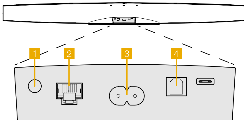
图1 Formation Bar 后面板
