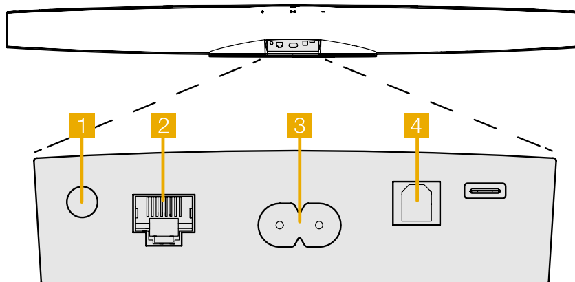
図 1 Formation Bar リアパネル
