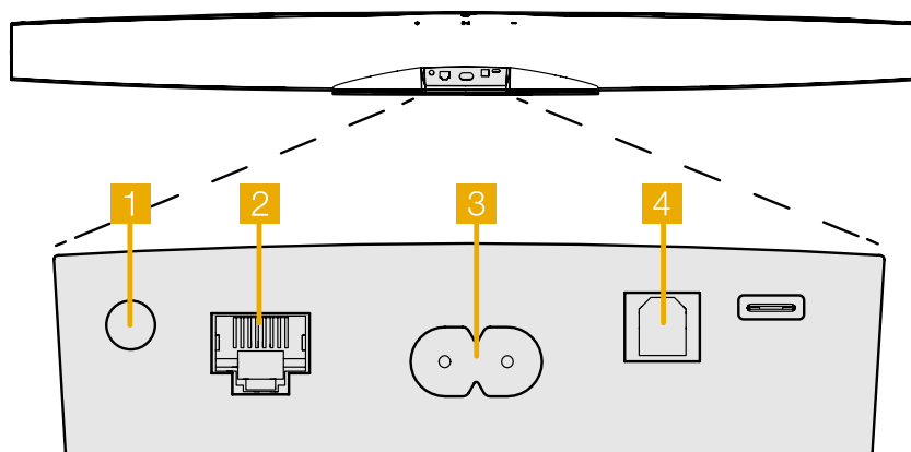
Obrázek 1 Zadní panel Formation Bar
